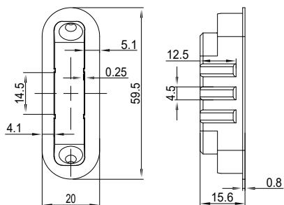
Ответная планка
