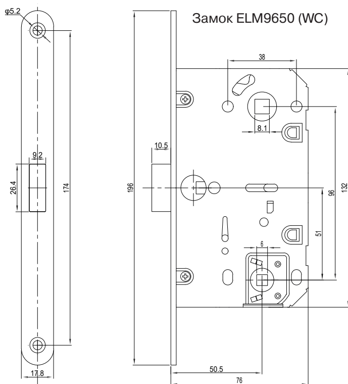
Ответная планка
