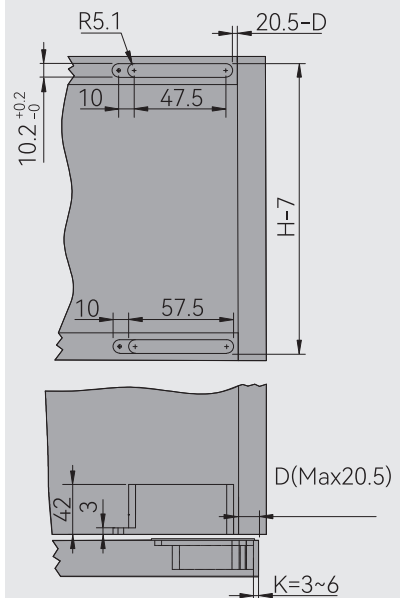
крепление петли в корпус без вставки
