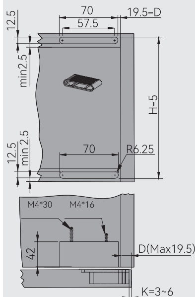
крепление петли в корпус с вставкой
