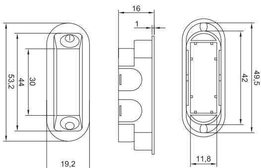
Ответная планка
