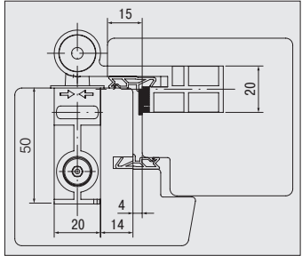
Створка с наплавом 15 мм и уплотнителем
