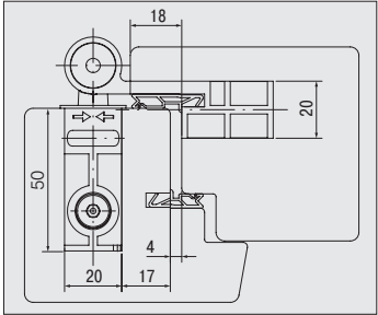
Створка с наплавом 18 мм и уплотнителем
