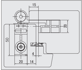
Створка с наплавом 15 мм
