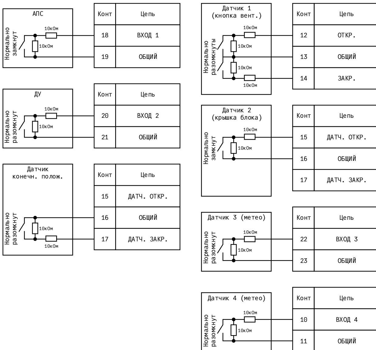
Рисунок 4 – Схемы подключения линий АПС, ДУ, Датчик конечного положения, Датчик 1, Датчик 2, Датчик 3, Датчик 4
