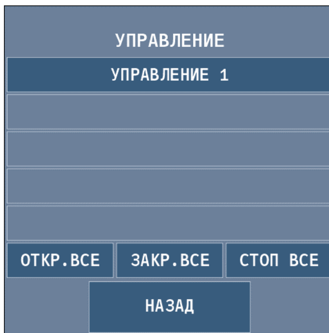
Рисунок 12 – Меню «Управление»
