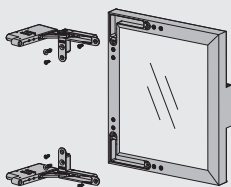
Регулировка по горизонтали
