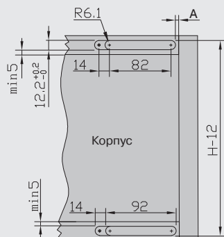
крепление петли в корпус без вставки
