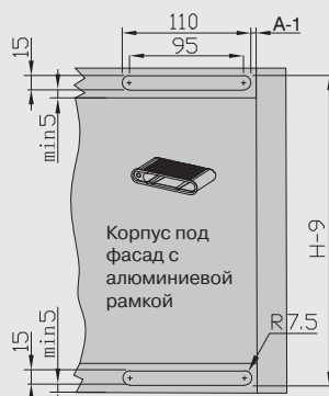
крепление петли в корпус с вставкой
