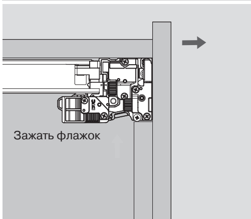
Зажмите флажок на фиксаторе и потяните ящик на себя
