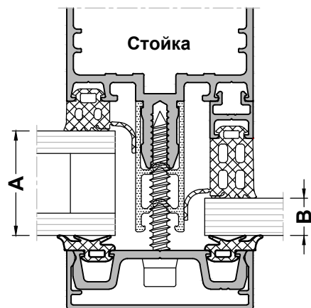
Наружный уплотнитель остекления ALM750004 (4 мм) или ALM750007 (6 мм)
