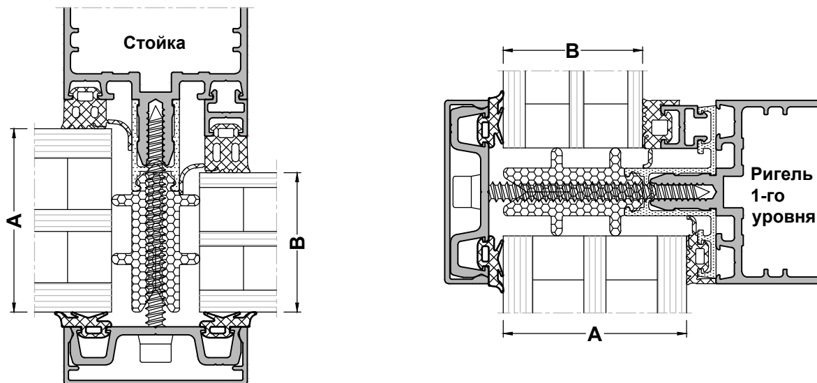
Наружный уплотнитель остекления ALM750004 (4 мм) или ALM750007 (6 мм)
