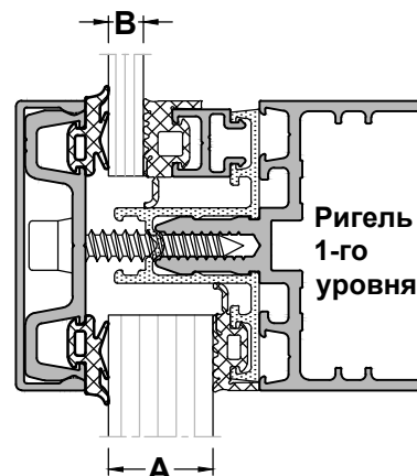
Наружный уплотнитель остекления ALM750004 (4 мм) или ALM750007 (6 мм)
