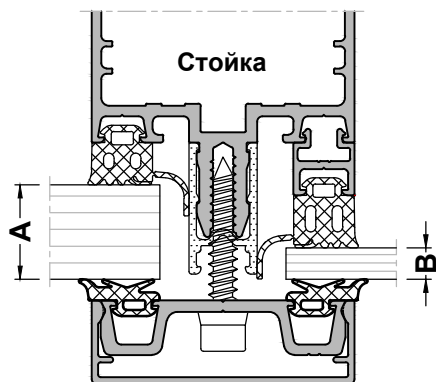
Наружный уплотнитель остекления ALM750004 (4 мм) или ALM750007 (6 мм)
